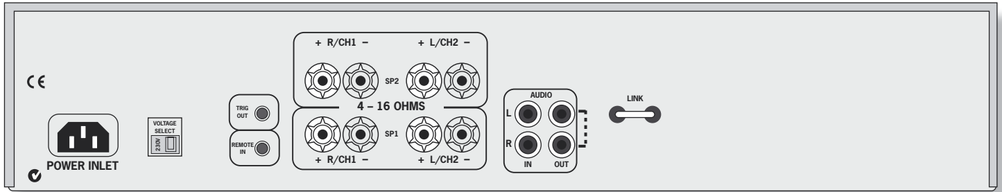
P35 Power Amplifier: rear panel
